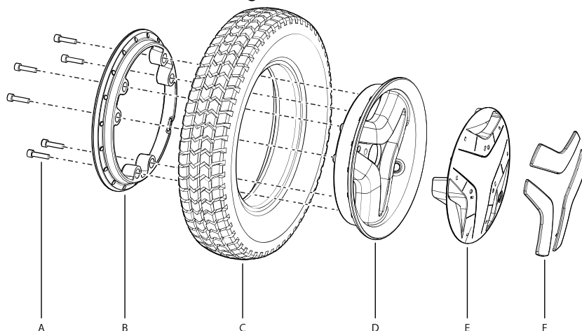
Abbildung 200. Anbringung oder Ausbau von Vollgummireifen oder Luftreifen.
