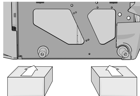
Abbildung 193. Verwenden Sie jeweils zwei Blöcke auf jeder Seite des Fahrgestellkastens. Zur besseren Darstellung wurden die Räder in dieser Abbildung entfernt.
