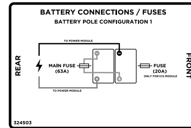
Abbildung 113. Batteriepole, Hauptschalter und Sicherung sind für Produkte mit 60 Ah-Batterien ausgelegt.
