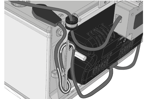
Abbildung 180. Schließen Sie das Kabel vom linken, hinteren Batteriepol am zugehörigen Kabelhalter an, siehe Abbildung.
