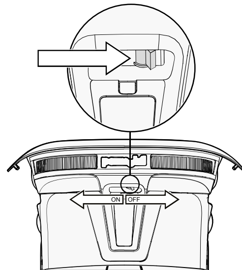
Abbildung 189. Hauptschalter unter dem Permobil-Logo auf der hinteren Abdeckung.
