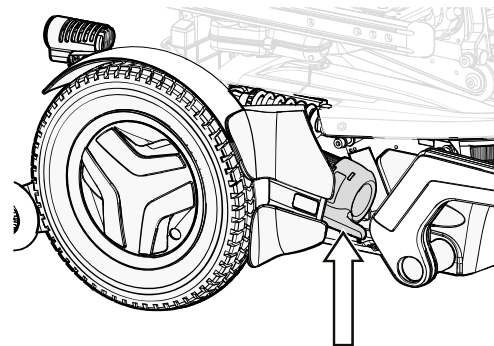
Abbildung 213. Bremsentriegelungshebel
