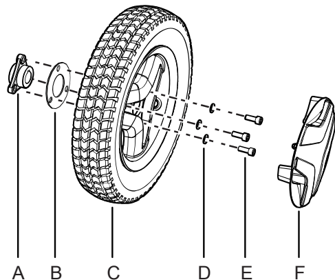
Abbildung 190. Montieren des Antriebsrads.
