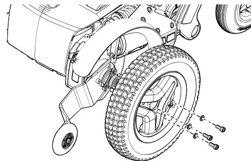
Abbildung 197. Bringen Sie das Rad auf der Radnabe an.
