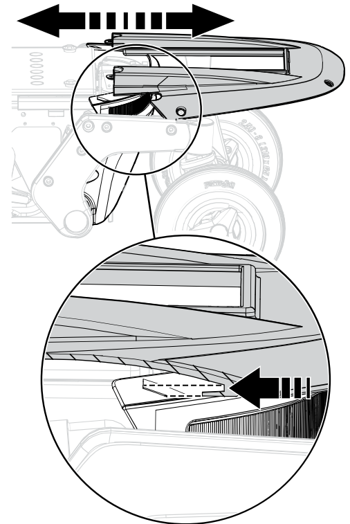
Abbildung 171. Obere Abdeckung.
