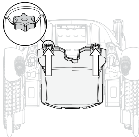
Abbildung 188. Die Abdeckungen des Fahrgestellkastens sind mit zwei Knäufen gesichert.
