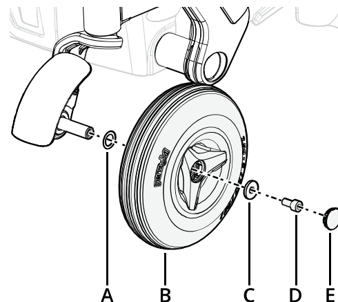
Abbildung 208. Zusammenbauen der Felge.
