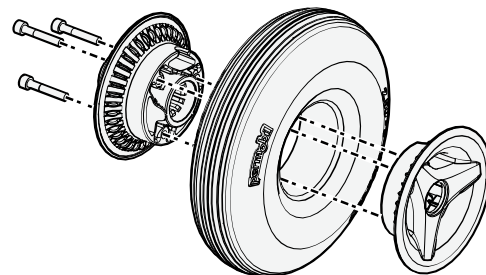
Abbildung 209. Felge.
