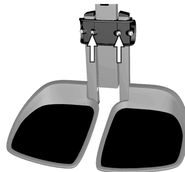
Abbildung 1.33. Einstellungsschrauben für die Beinstützenlänge.
