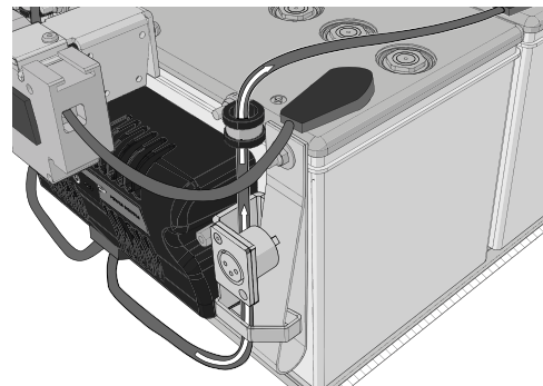
Abbildung 181. Schließen Sie das Kabel vom rechten, vorderen Batteriepol am zugehörigen Kabelhalter an, siehe Abbildung.
