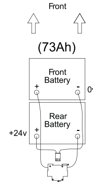
Abbildung 179. Schaltplan für den Batterieanschluss.
