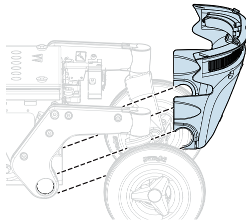
Abbildung 172. Hintere Abdeckung.
