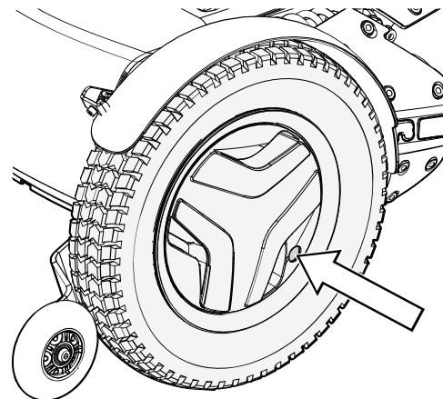
Abbildung 201. Luftventil am Antriebsrad
