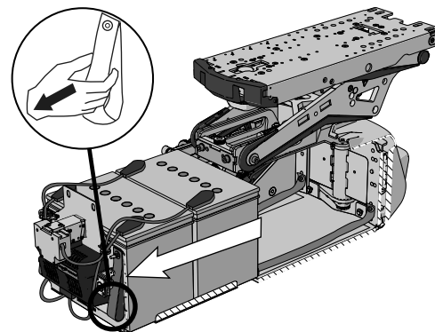
Abbildung 176. Bänder zum Herausziehen des Batteriekastens.
