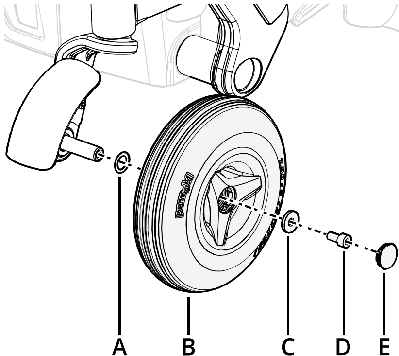
Abbildung 202. Zusammenbauen der Felge.
