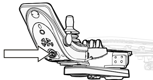
Abbildung 17. Ladesteckdose.
