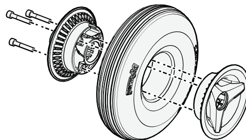
Abbildung 210. Felge.
