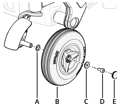
Abbildung 207. Zusammenbauen der Felge.
