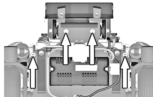
Abbildung 174. Der Batteriekasten ist mit vier Schrauben befestigt.
