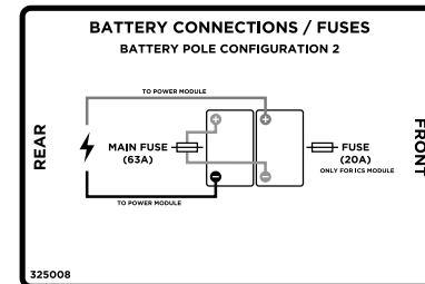
Abbildung 114. Batteriepole, Hauptschalter und Sicherung sind für Produkte mit 73 Ah-Batterien ausgelegt.
