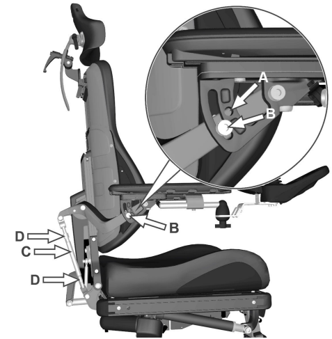
Abbildung 131. Einstellung von Armlehnenhöhe und -winkel.
