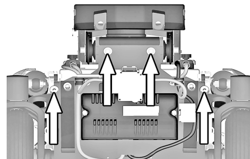
Abbildung 184. Der Batteriekasten ist mit vier Schrauben befestigt.
