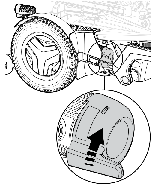
Abbildung 151. Aktivieren der Radsicherungen.
